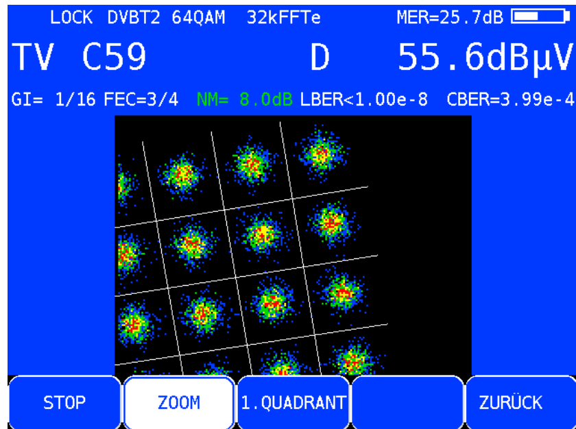
Konstellationsdiagramm DVB-T2 Zoom
