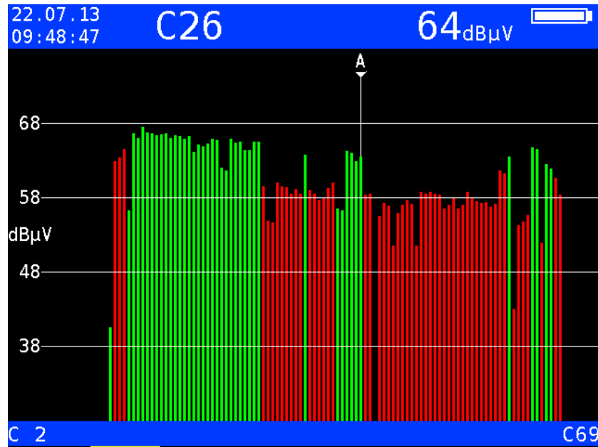
Pegeldiagramm
