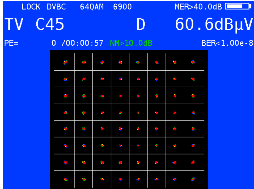
Ideales Konstellationsdiagramm
