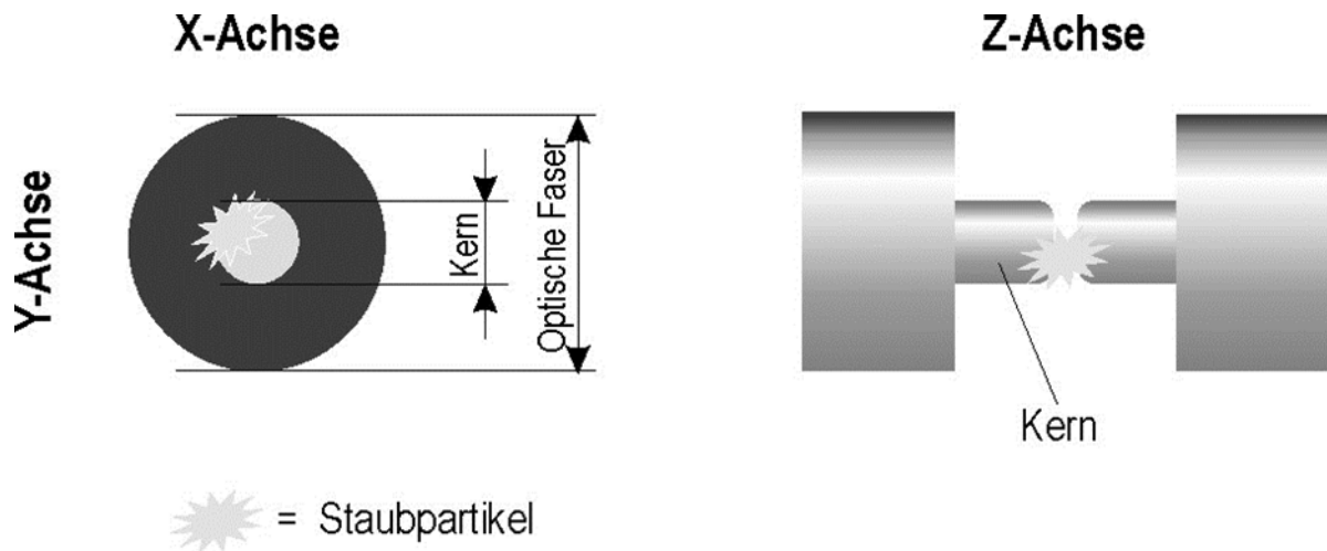
Schlechter physikalischer Kontakt durch Staubpartikel
