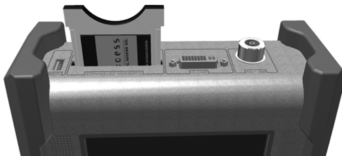
Einsetzen eines CA-Moduls
