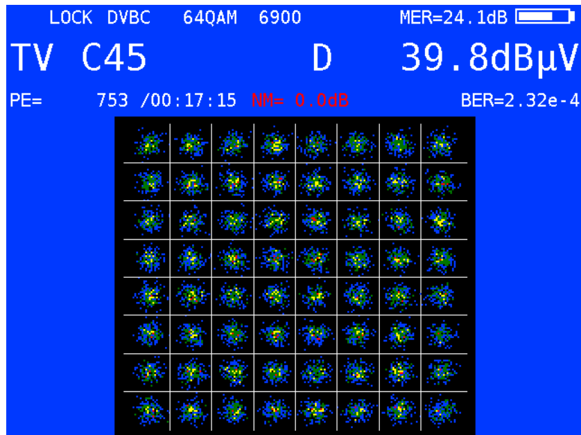
Konstellationsdiagramm mit verrauschtem Signal
