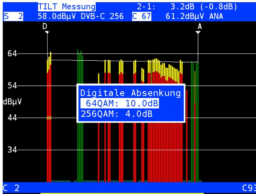
Schräglagenmessung Einstellung der Pegelabsenkung
