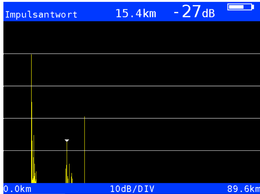
DVB-T2 Impulsantwort
