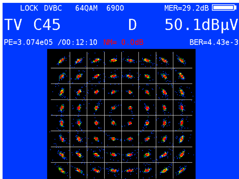
Konstellationsdiagramm mit Phasenjitter
