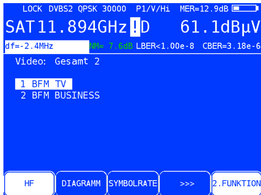
Frequenzoffset anzeigen
