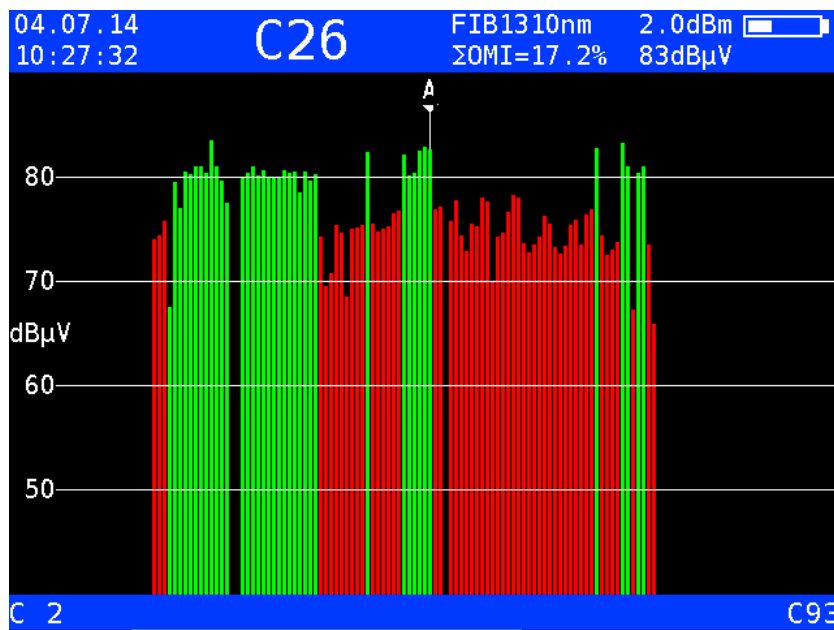
Analyzerbild mit Summen-OMI
