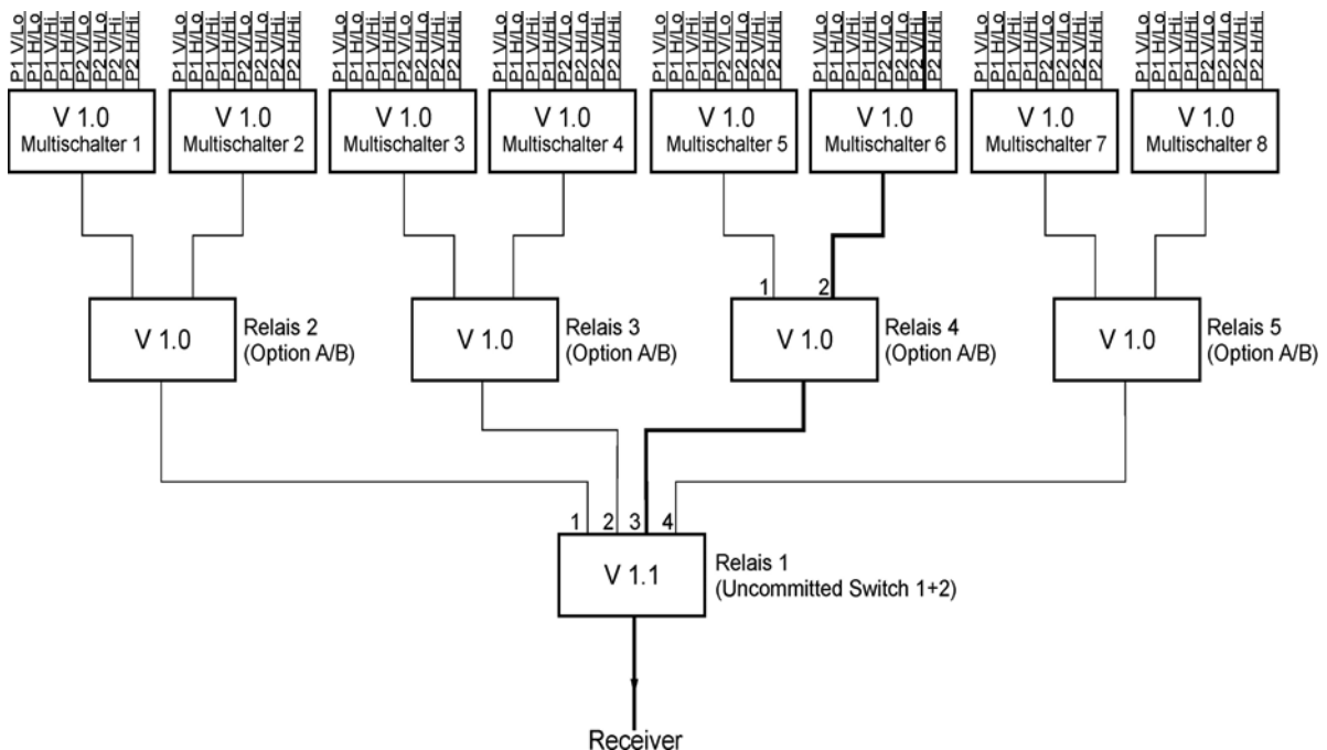
DiSEqC V1.1 Aufbau mit 64 SAT-ZF Ebenen
