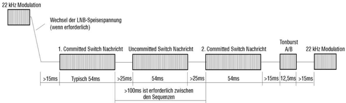
DiSEqC V1.1 Steuerablauf mit Wiederholung
