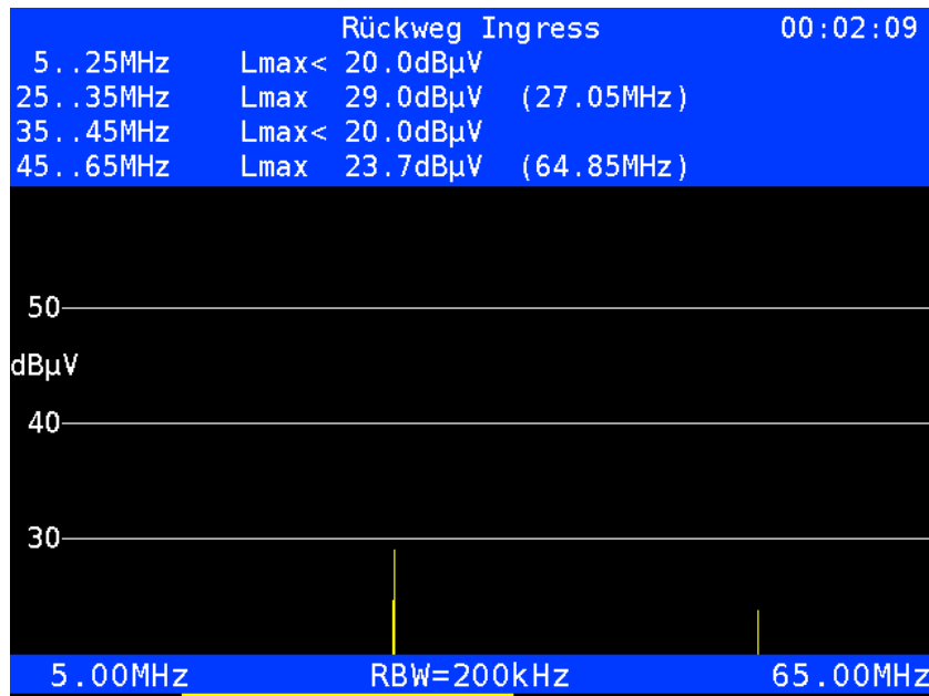
Spektrumanalyzer Ingressmessung
