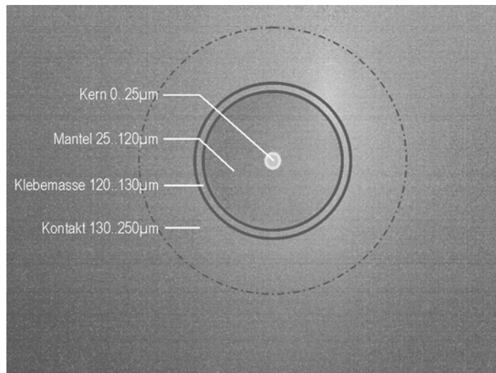
Kernaufbau einer Singlemode-Faser
