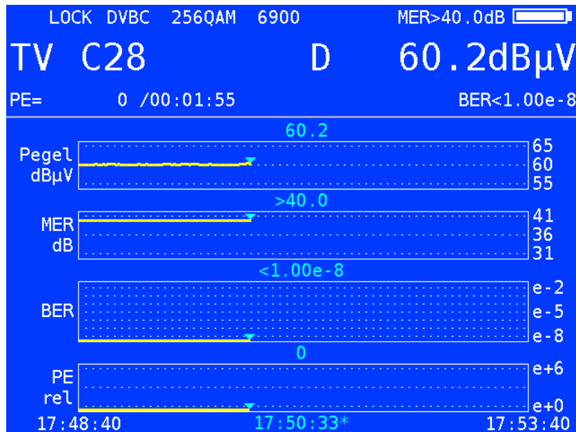
DataGrabber Aufzeichnung
