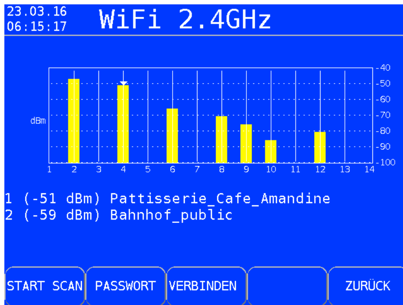
WLAN Kanaldiagramm
