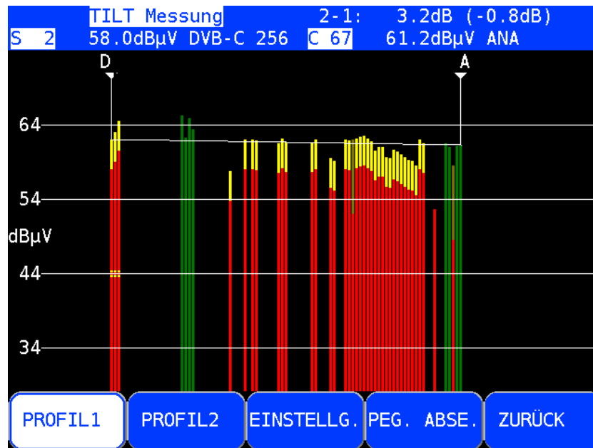
Schräglagenmessung TILT
