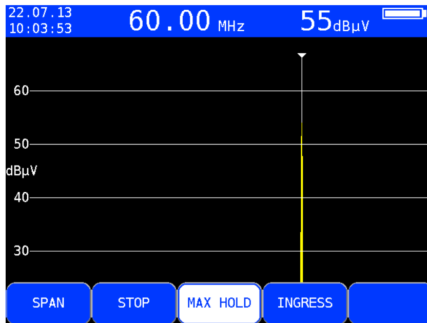
Spektrumanalyzer Max-Hold Funktion
