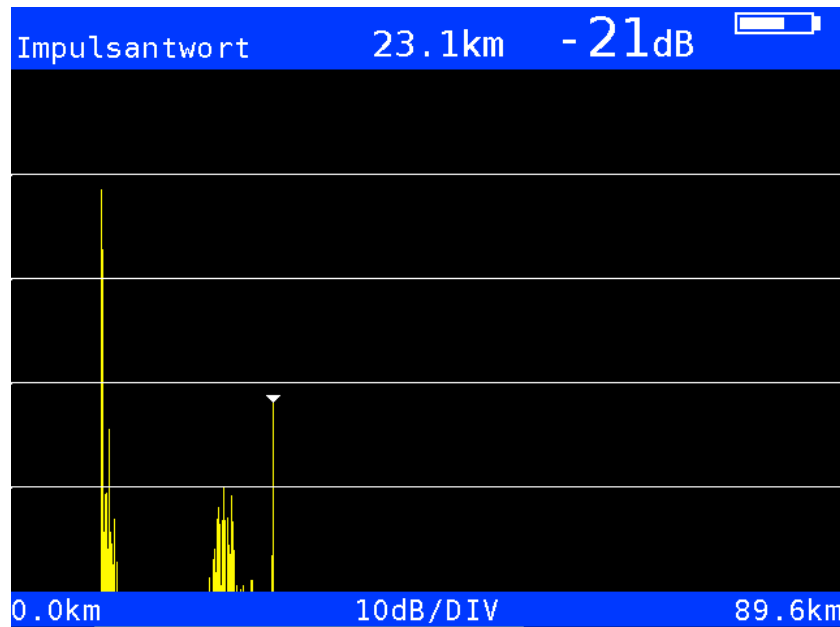
DVB-T Impulsantwort
