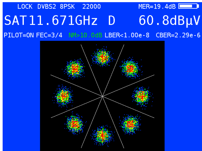
DVB-S2 Konstellationsdiagramm
