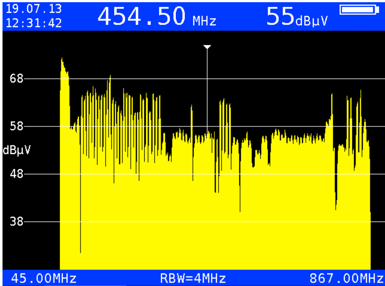
Spektrumanalyzer: Spektrum Breitbandkabel
