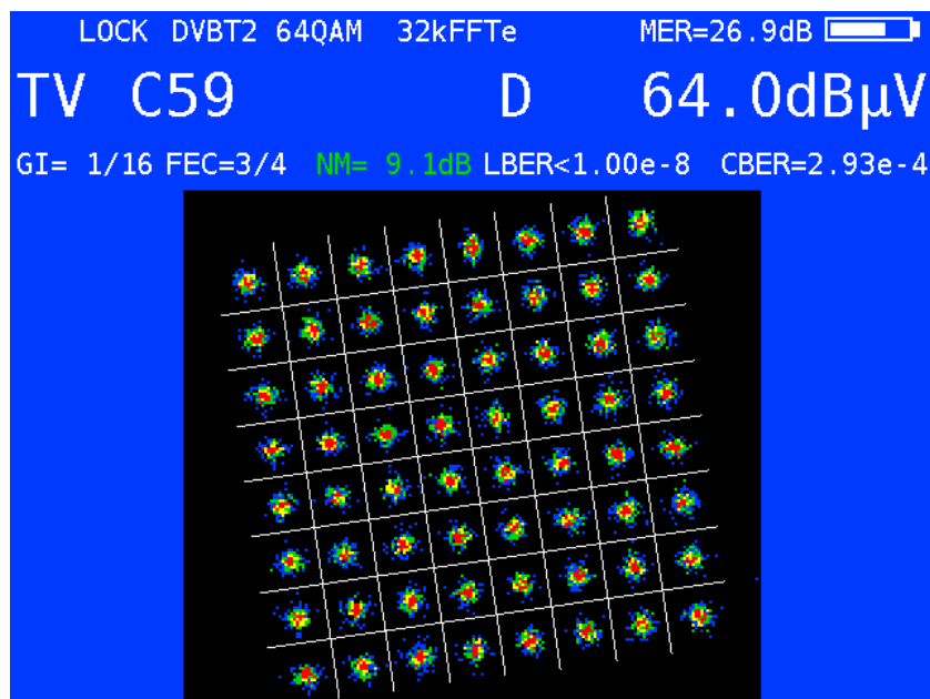
Reales Konstellationsdiagramm DVB-T2
