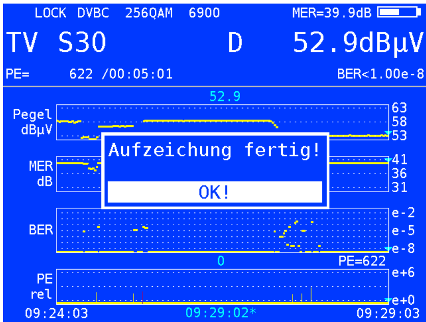
DataGrabber Aufzeichnung Ende
